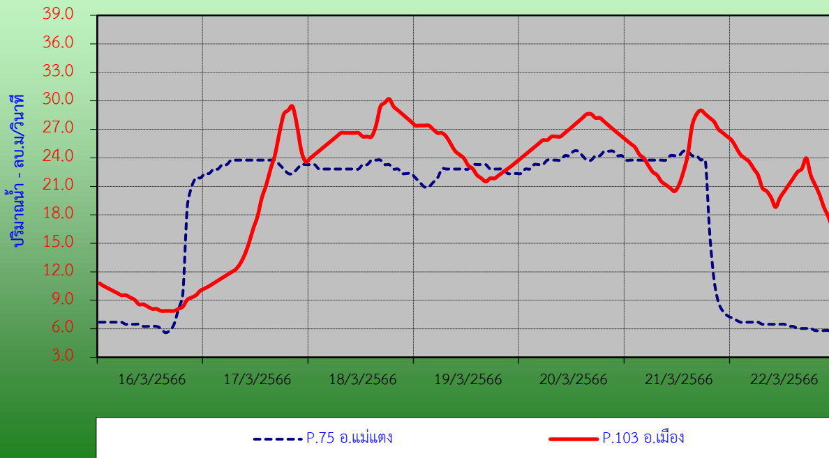
กราฟแสดงปริมาณน้ำปิงรายชั่วโมงรอบวันที่ 11/2566 ที่สถานีแม่ น้ำปิง ( P.75) บ้านซ้อแล อ.แม่แตง และที่สถานีแม่ น้ำปิง (P.103) บ้านป่าซ่อยใต้ อ.เมือง จ.เชียงใหม่
